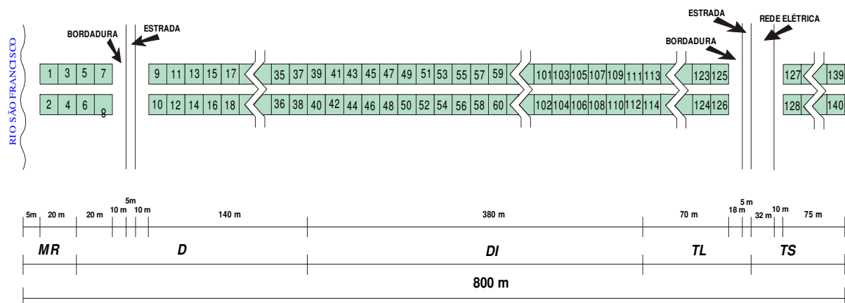
Anexo 2 - Projeção horizontal do transecto com implantação das 140 parcelas no remanescente de caatinga à margem do rio São Francisco. EMBRAPA-SPSB, Petrolina-PE.
