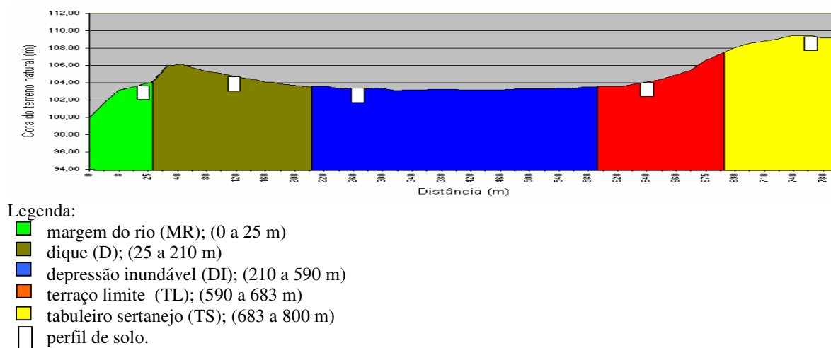
Figura 1 - Representação esquemática do perfil topográfico com a distribuição dos cinco ambientes topográficos e dos perfis de solo no remanescente de caatinga à margem do rio São Francisco. EMBRAPA-SPSB, Petrolina-PE.
